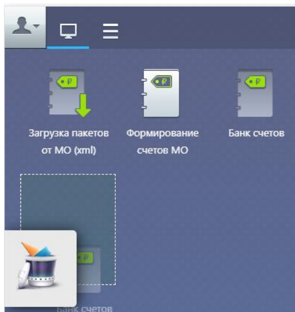
Рисунок 9 – Удаление ярлыка
