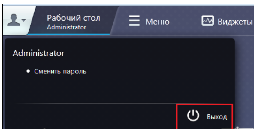
Рисунок 3 – Кнопка «Выход»
