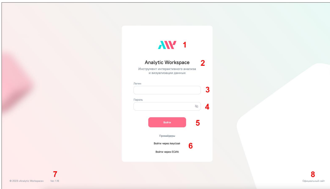
Рисунок 49 – Окно авторизации
